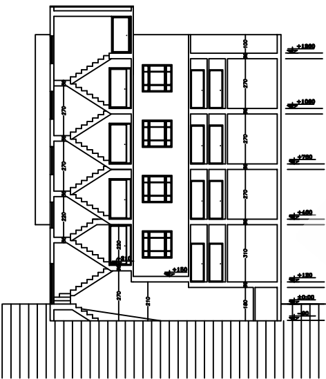
SECTION A-A SC. 1:100
