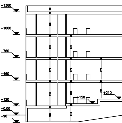
مقطع B-B Scale 1:100
