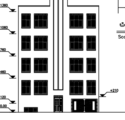
نمای شمالي Scale 1:100
