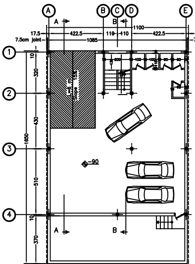
پلان زير زمين Scale 1:100
