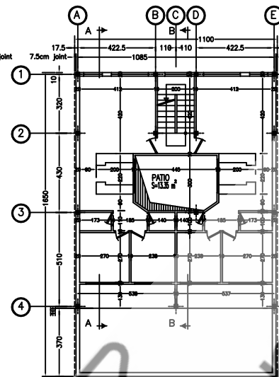
پلان طبقه ۳، ۲، ۱ Scale 1:100
