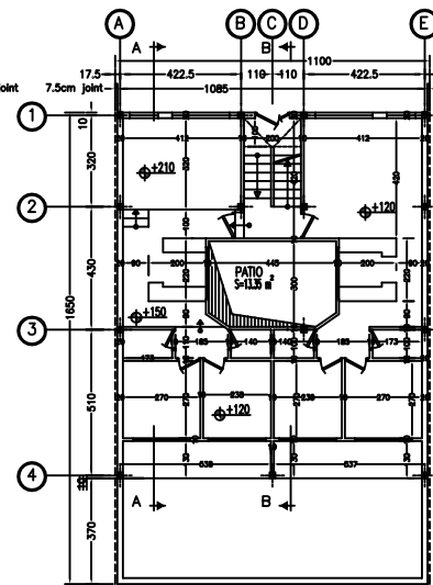
پلان طبقه همگف Scale 1:100
