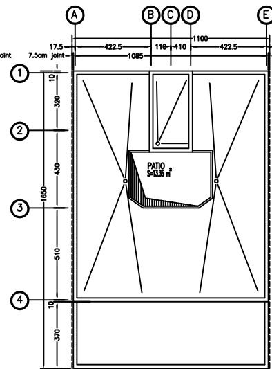
پلان باغ Scale 1:100
