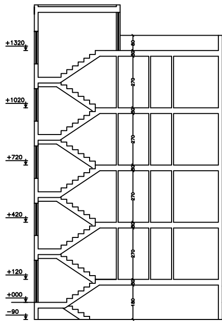
SECTION A-A SCALE 1:100
