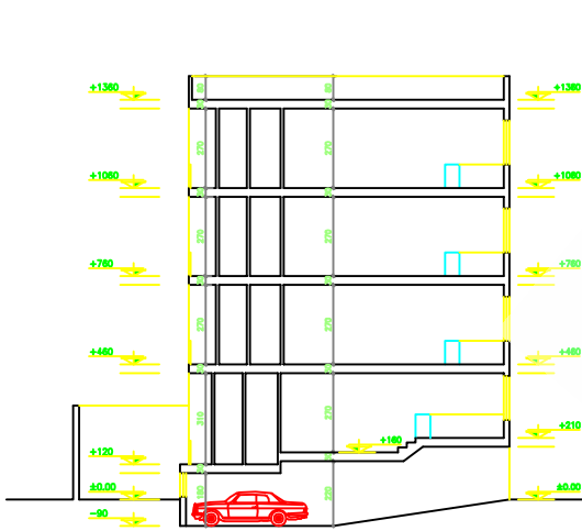
SECTION A-A SC. 1:100
